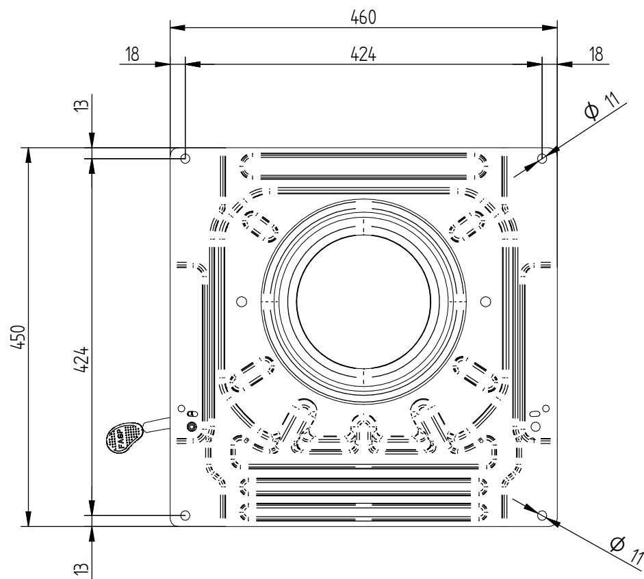
VISTA SUPERIORE
